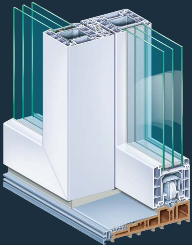
PremiDoor 88 Profilsystem für Hebe-Schiebetüren Bautiefe Flügel: 88 mm, Zarge: 207 mm
