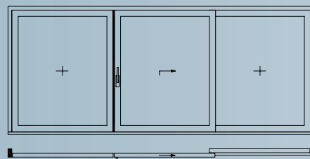
Schema G-A 3-teilig mit einem Hebe-Schiebeflügel und zwei Festverglasungen
