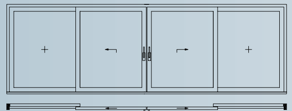
Schema C 4-teilig mit zwei Hebe-Schiebeflügeln und zwei Festverglasungen
